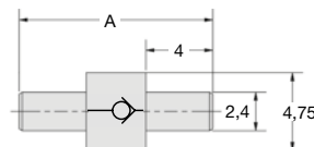
F2804-40.-mit glattem Nippel
